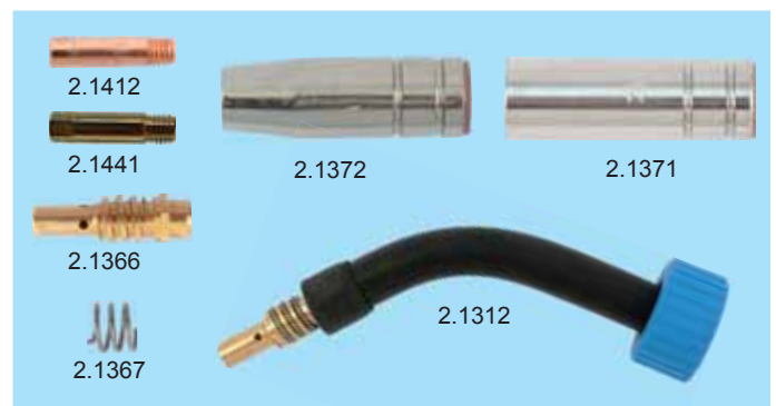
Komplettbrenner sind bei Lieferung ausgerüstet für Stahldraht 0,8 mm.
